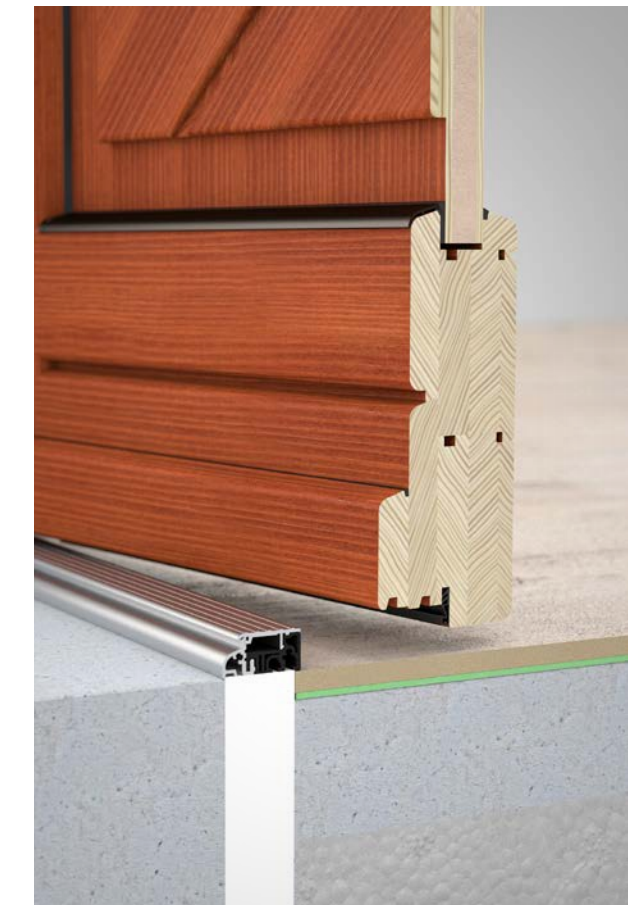
Próg standardowy.
