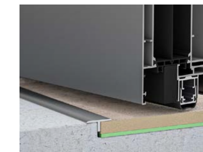
Próg z automatyczną uszczelką.
